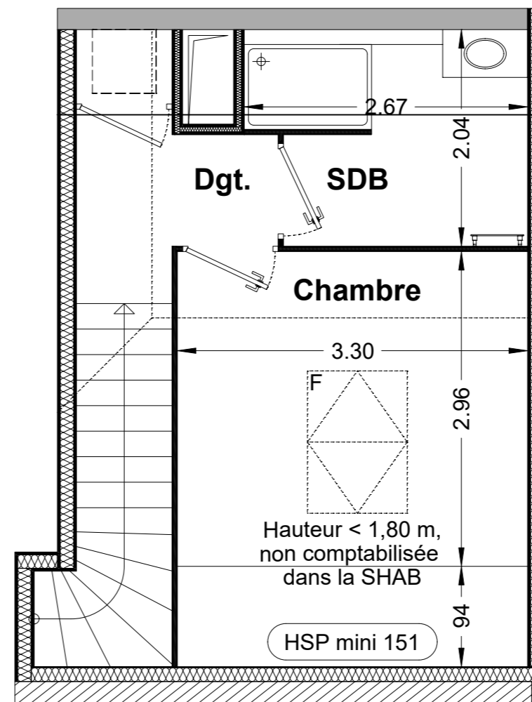
PLAN DES COMBLES
