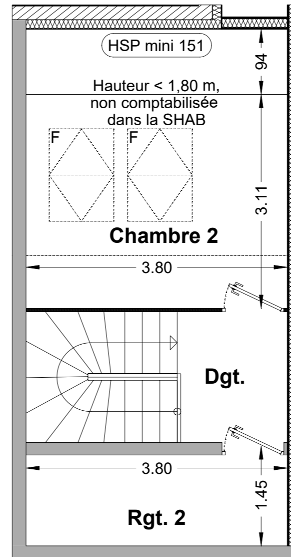
PLAN DES COMBLES
