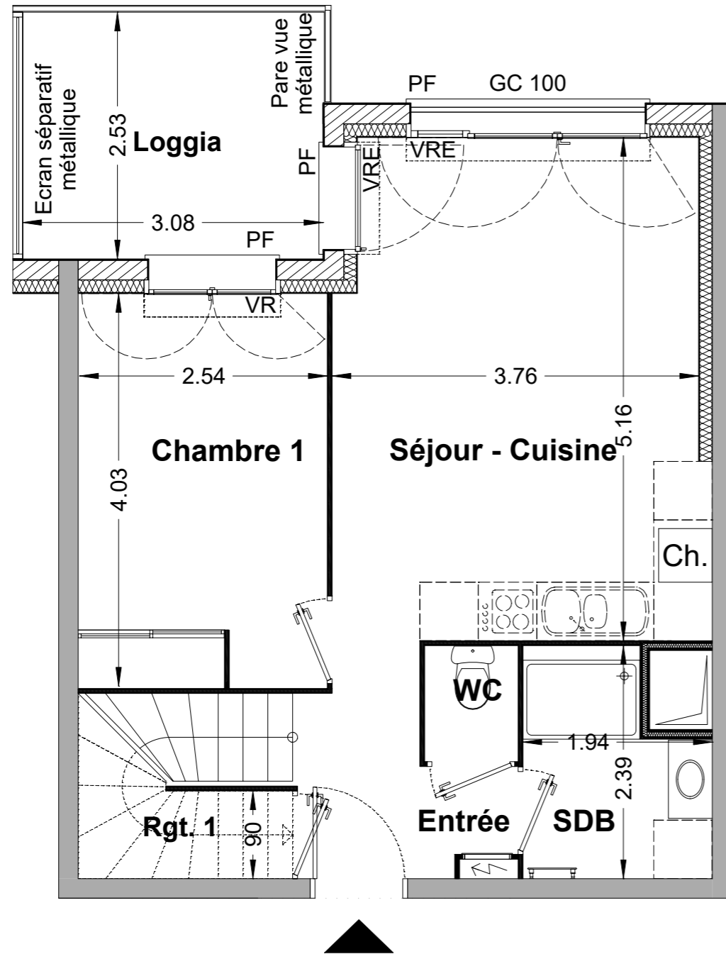
PLAN DU R+1
